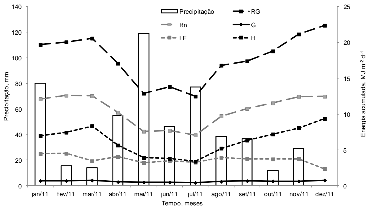
Figura 11 - Total mensal da precipitação pluvial e média mensal dos fluxos de radiação (Rg) e energia (Rn, LE, H e G) em Brachiaria decumbens no município de São João, PE
